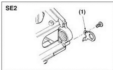
(1) Петля подвеса
