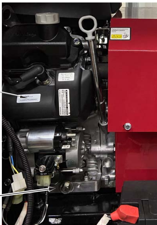
ЗАВОДСКОЙ НОМЕР ДВИГАТЕЛЯ
