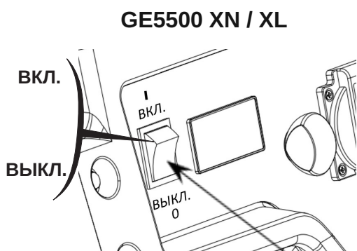
ВЫКЛЮЧАТЕЛЬ ДВИГАТЕЛЯ
